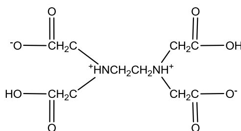
H_4EDTA (zwitterion)
