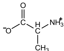
alanine (zwitterion notation)
