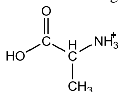
alaninium ion
