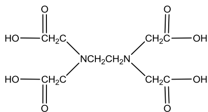
\text{H}_4\text{EDTA}
